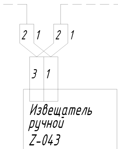
Рисунок 2.3 – Схема подключения базы извещателя
