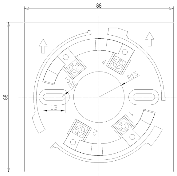
Рисунок 2.2 – Установочные размеры извещателя
